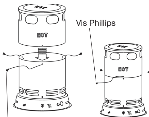
Vis de Support en Place
